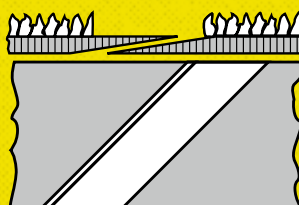
Forma 5 Slepeno s přesahem. Zóna zrna plně zbrúšena. Použití na bruskách s plochou kontaktní botkou, umožňuje jemný přechod oblasti pásového spoje.
