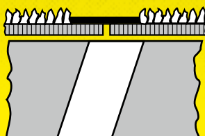
Forma 6 G Šikmý řez. Tupé spojení, slepené fólií zesílenou vláknem na straně zrna. Zóna zrna plně zbrúšena. Použití v průmyslovém opracování dřevěných materiálů.
