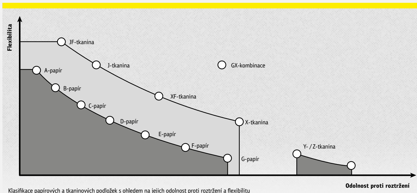
Klasifikace papírových a tkaninových podložek s ohledem na jejich odolnost proti roztržení a flexibilitu
